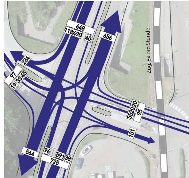
Abbildung 17: Knotenströme ASP inkl. Neuverkehr
