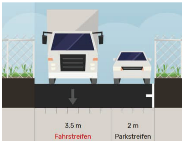
Abbildung 11: Querschnitt Steinibachweg [streettuner.fvv.tuwien.ac.at]
