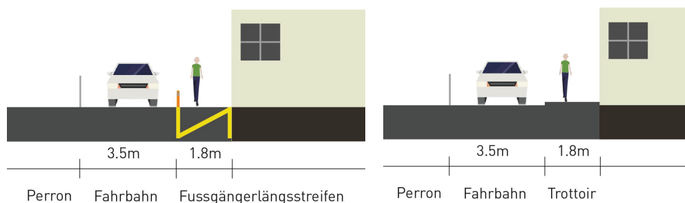
Abbildung 20: Gestaltungsvarianten Engstelle Hübeliweg [streettuner.fvv.tuwien.ac.at]
