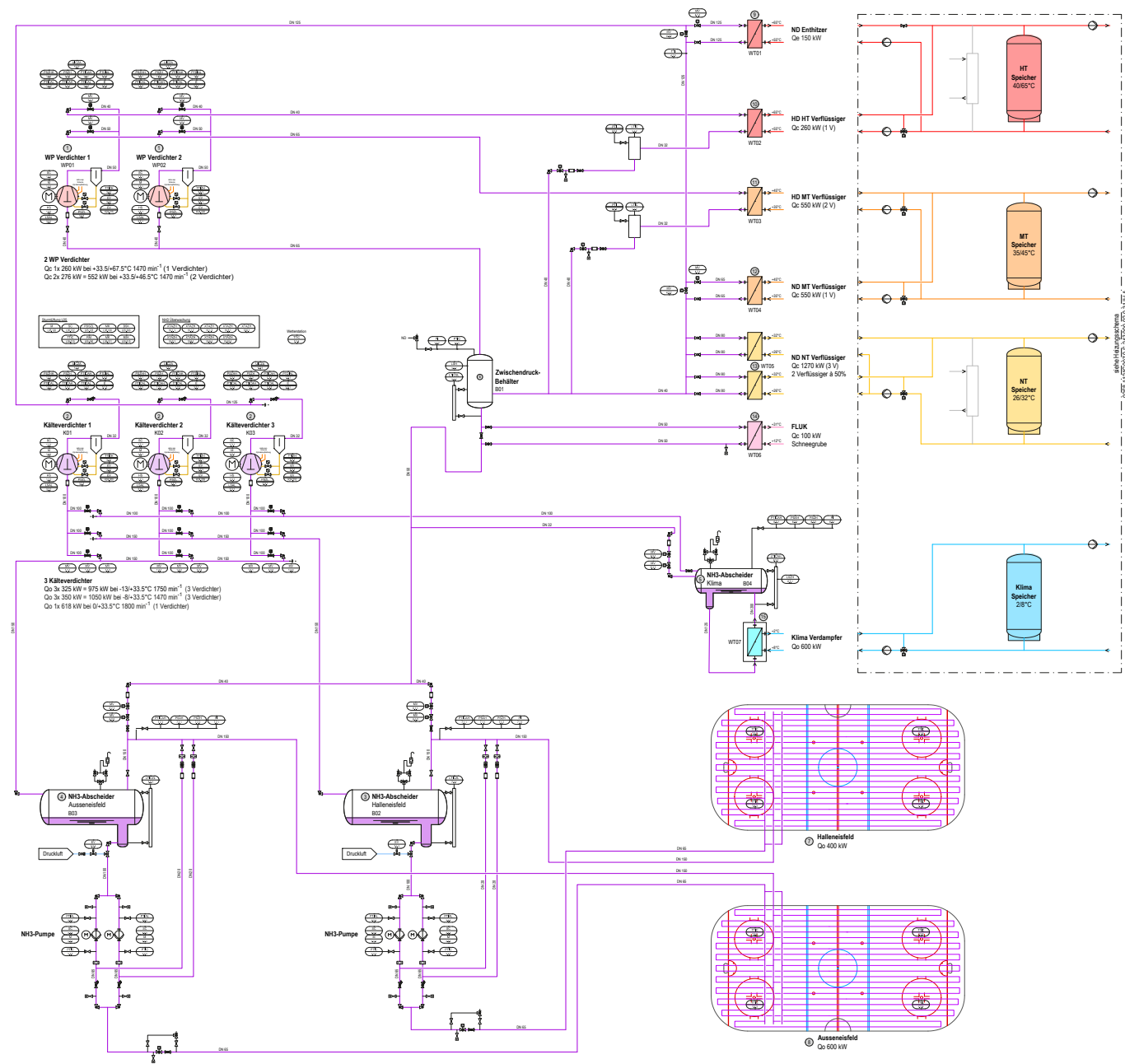
Schema Kälte
