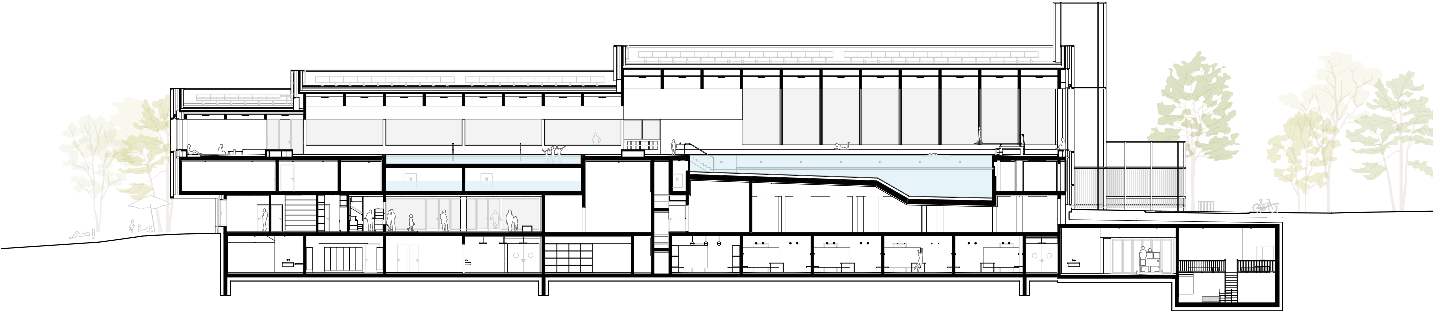
Längsschnitt Hallenbad
