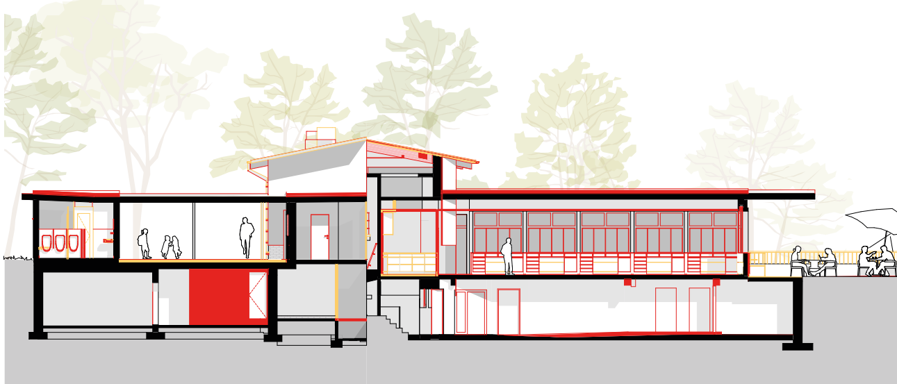
Längsschnitt
