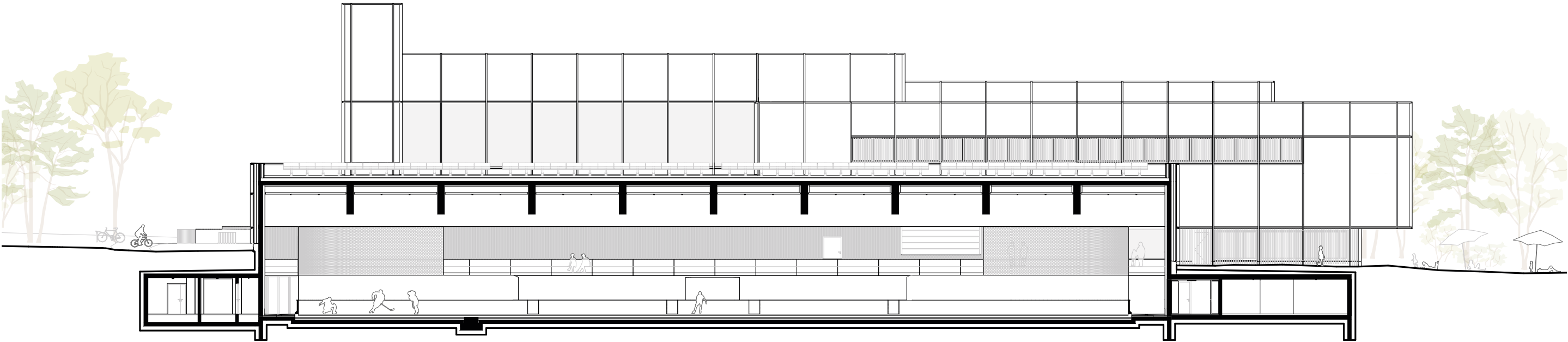
Längsschnitt Eishalle
