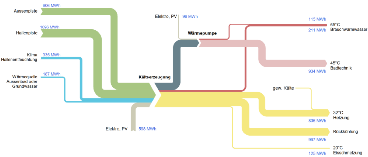
Jahres-Energieflussdiagramm
