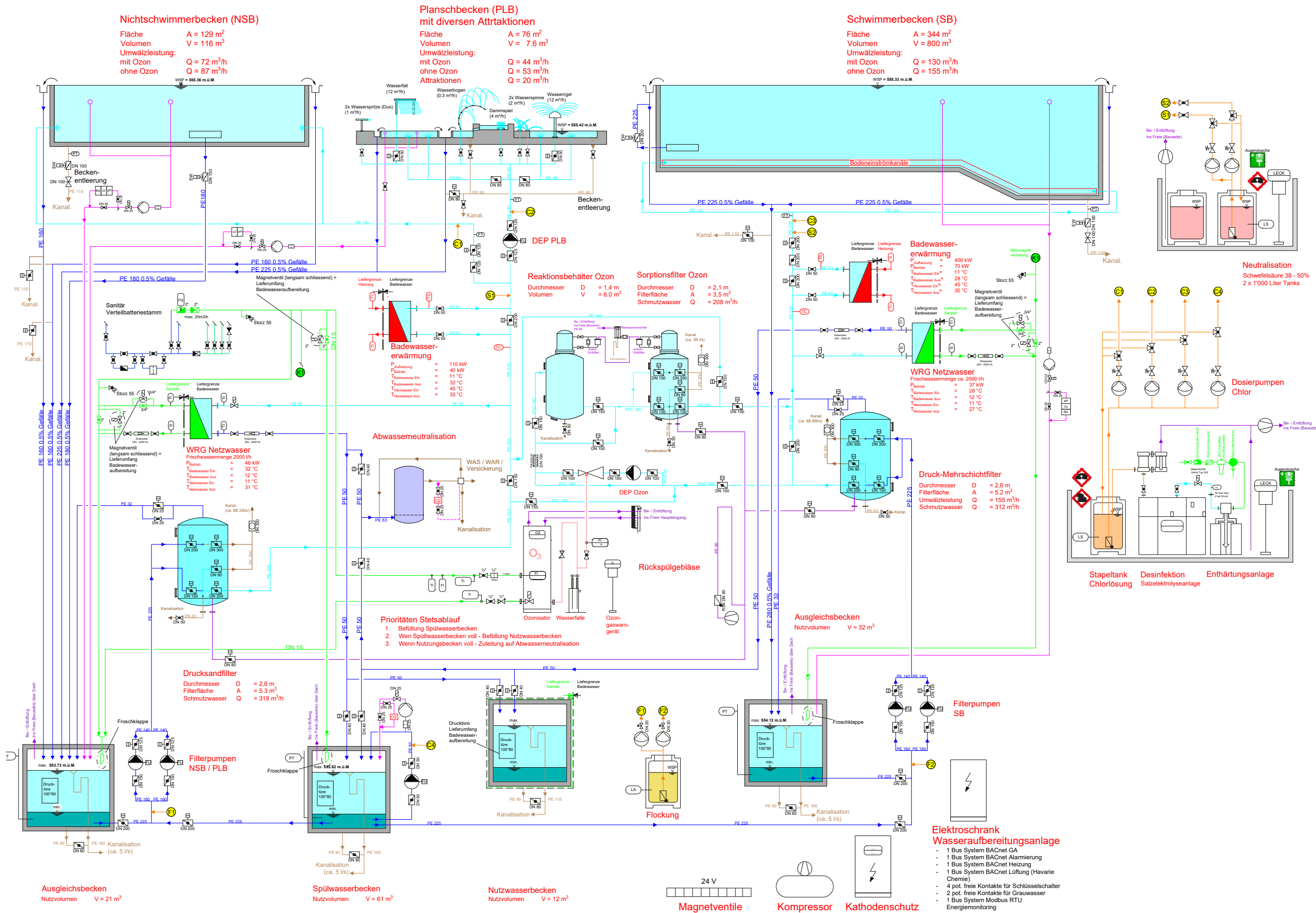
Schema Badewasseraufbereitung
