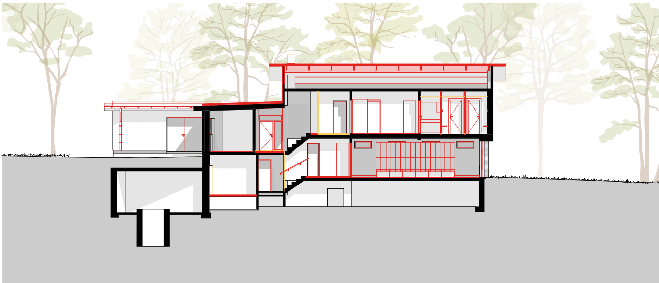
Querschnitt
