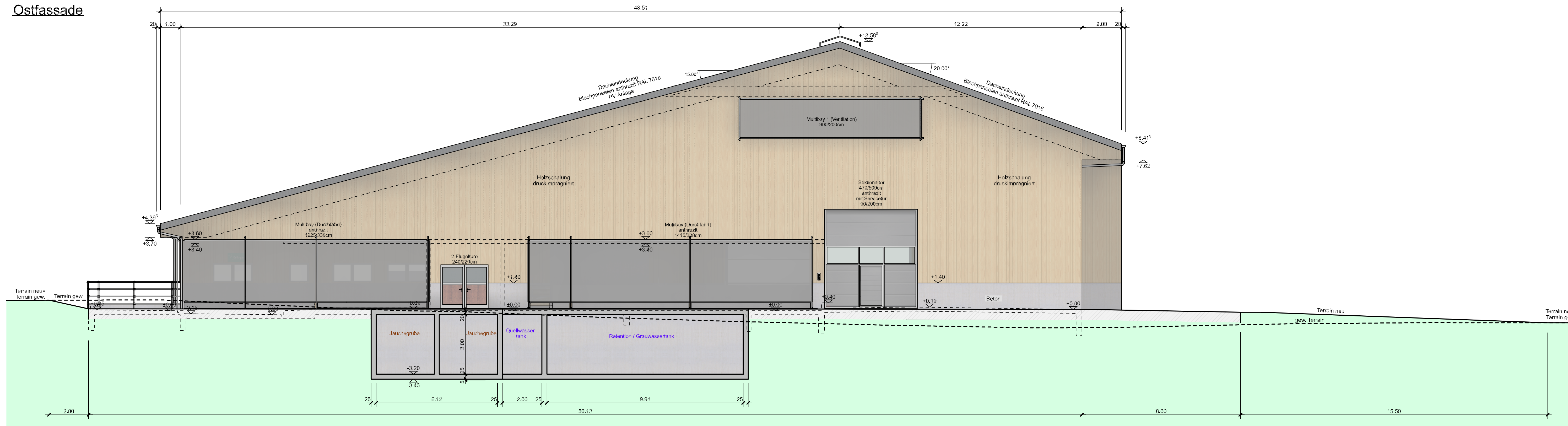
Südfassade
