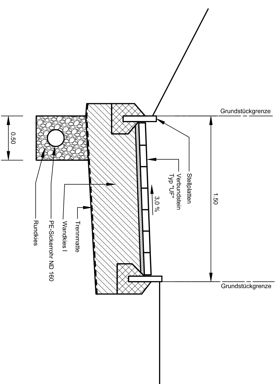
Normalprofil 1 - 1 1:20
