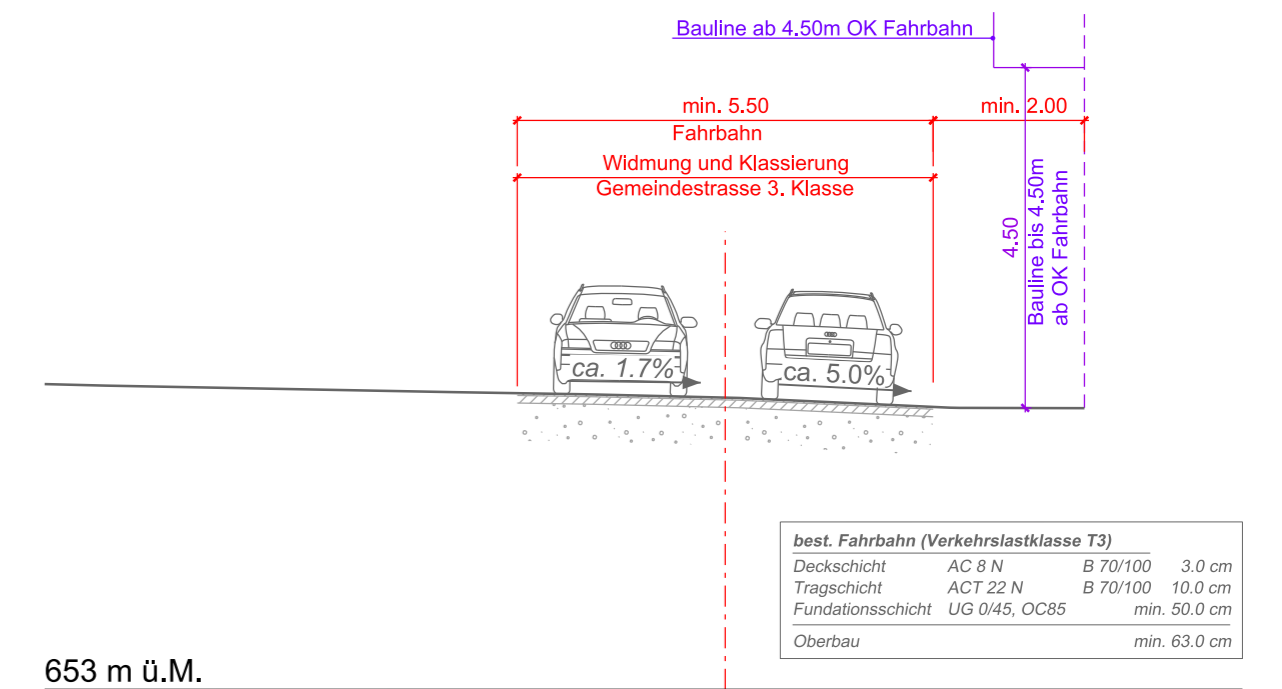
Querprofil 4 3+31.644
