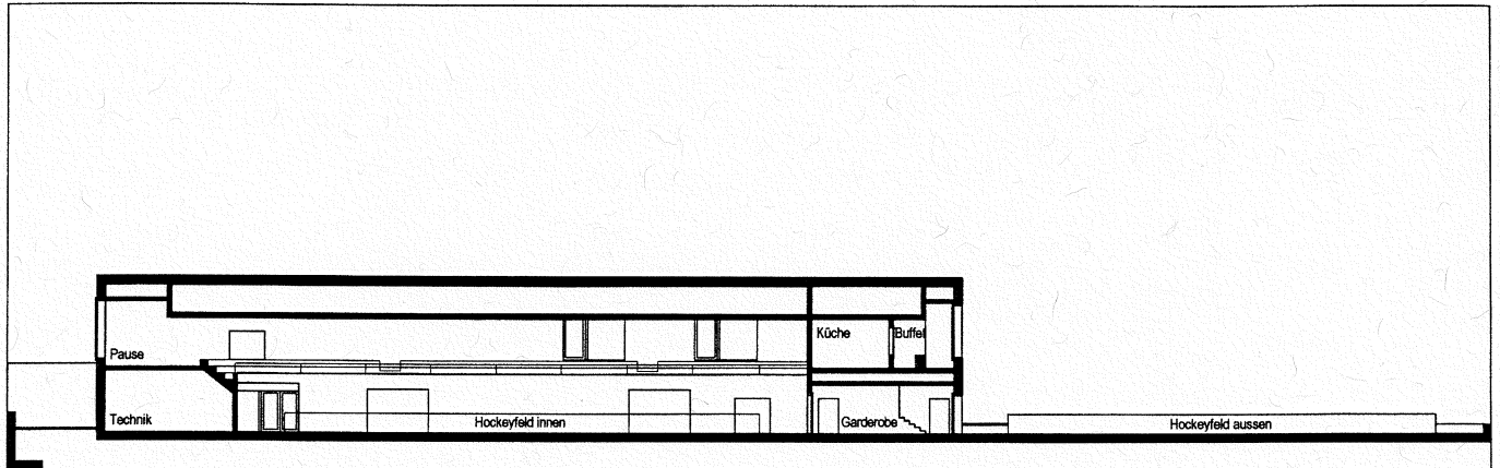
Querschnitt 1-1
