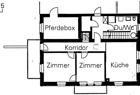
Erdgeschoss Projekt
