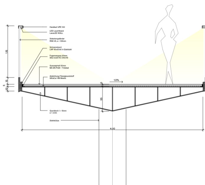
Querschnitt 1:20
