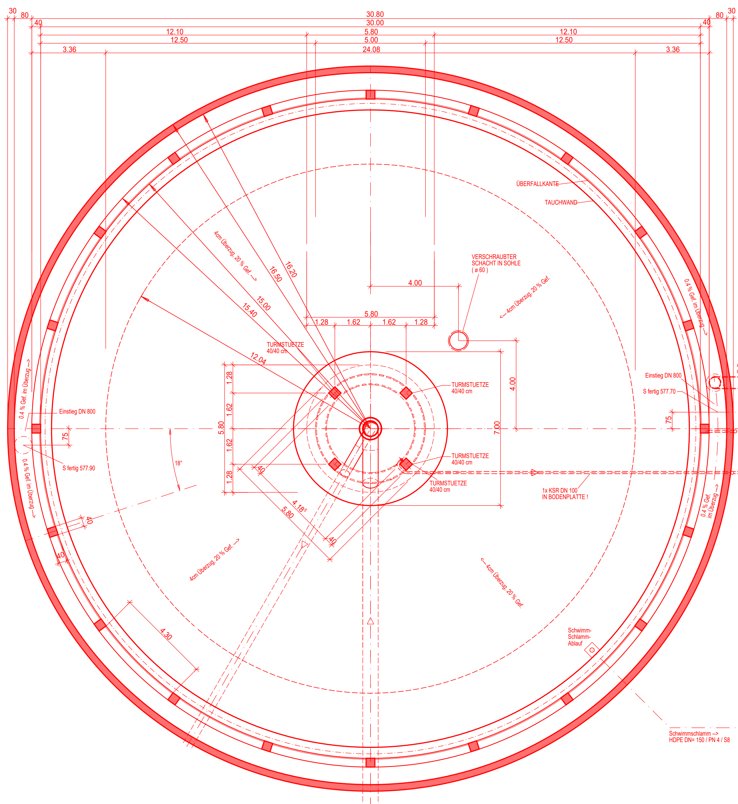
GRUNDRISS 2-2 1 : 100
