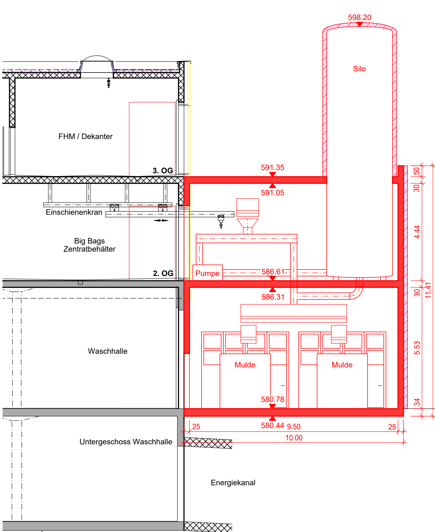
SNITT A-A
