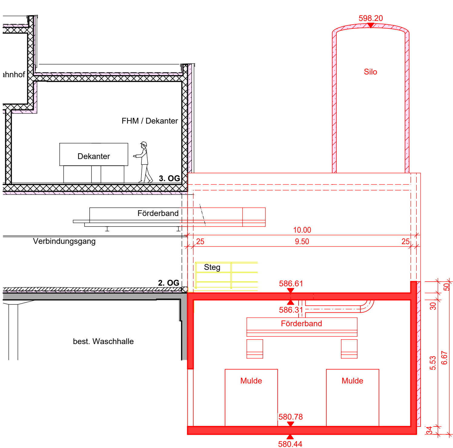
SNITT B-B
