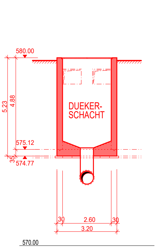
SNCHTT F-F 1 : 100
