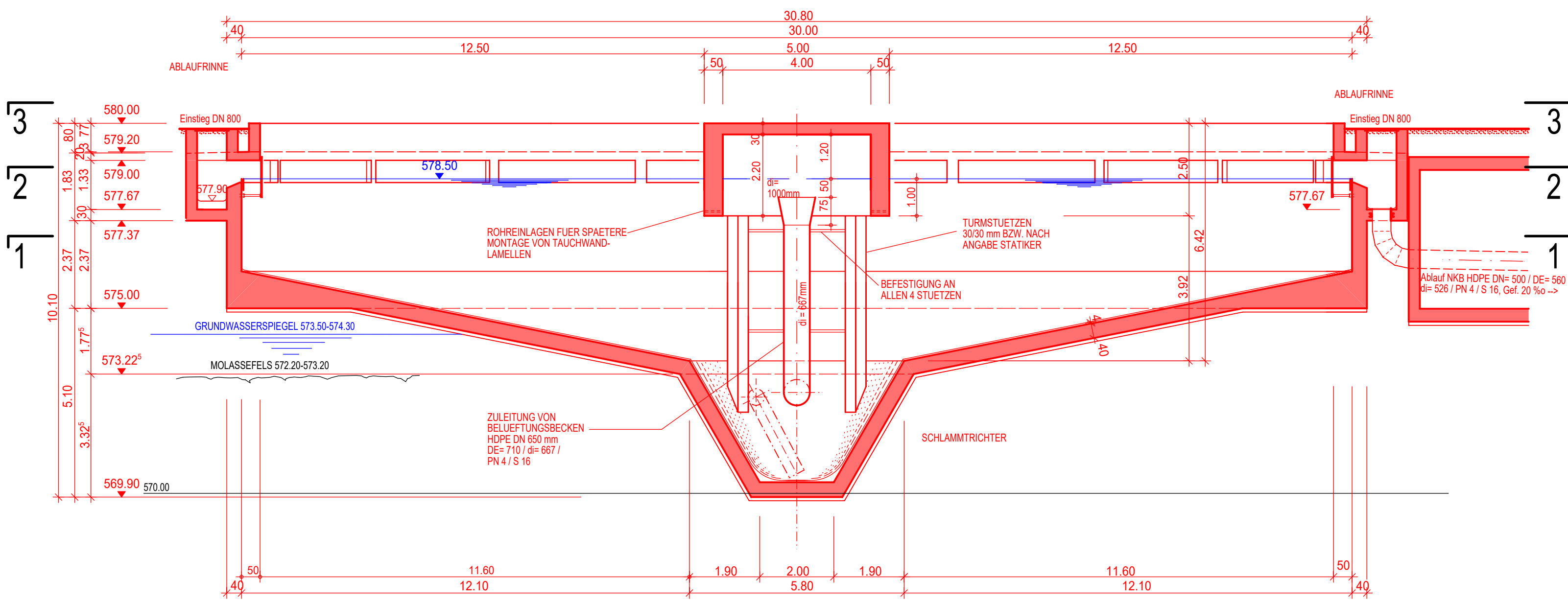
SNITT A-A 1 : 100
