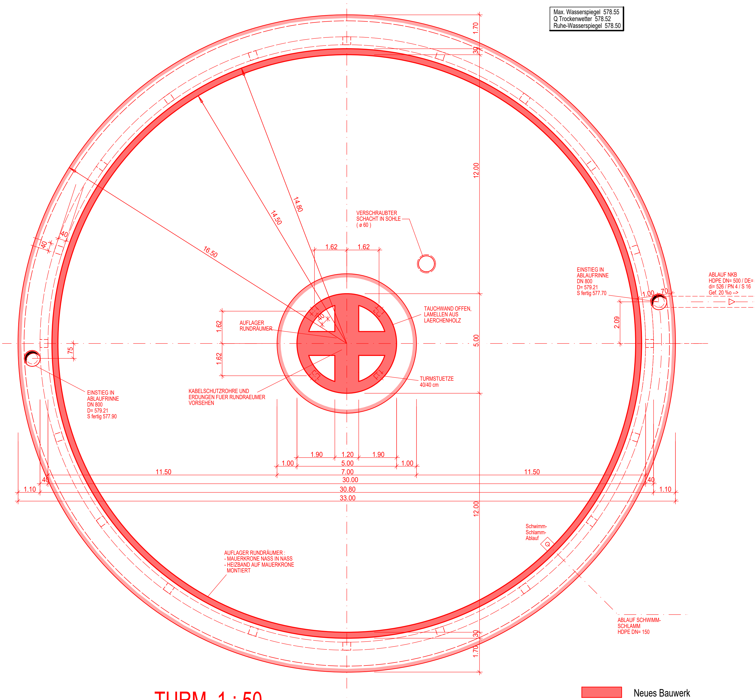
TURM 1 : 50 DRAUFSICHT
