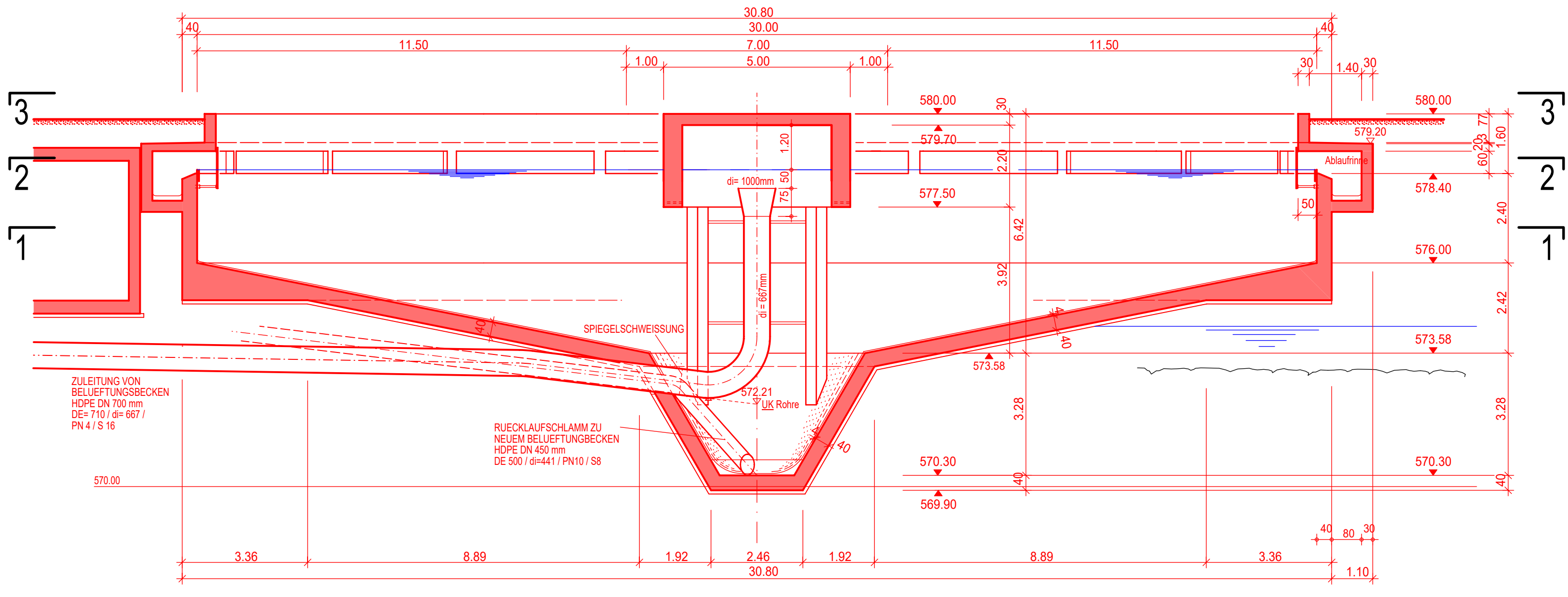
SNITT B-B 1 : 100
