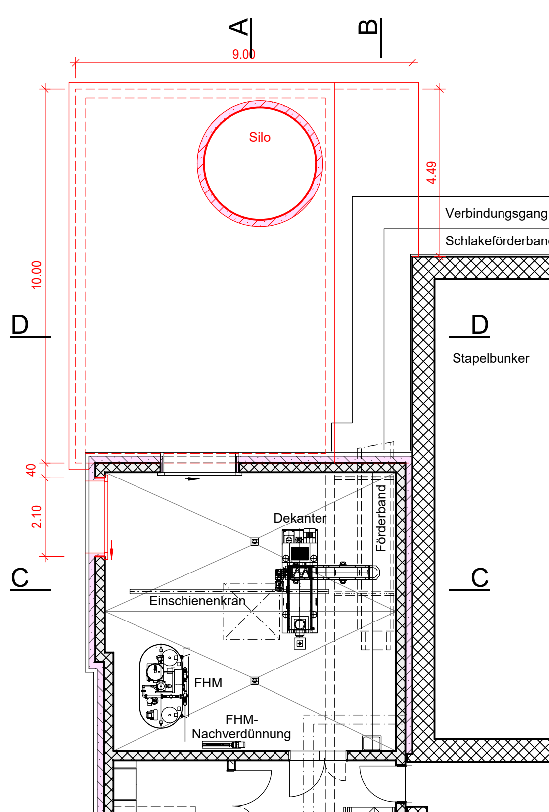
GRUNDRISS 3. OG
