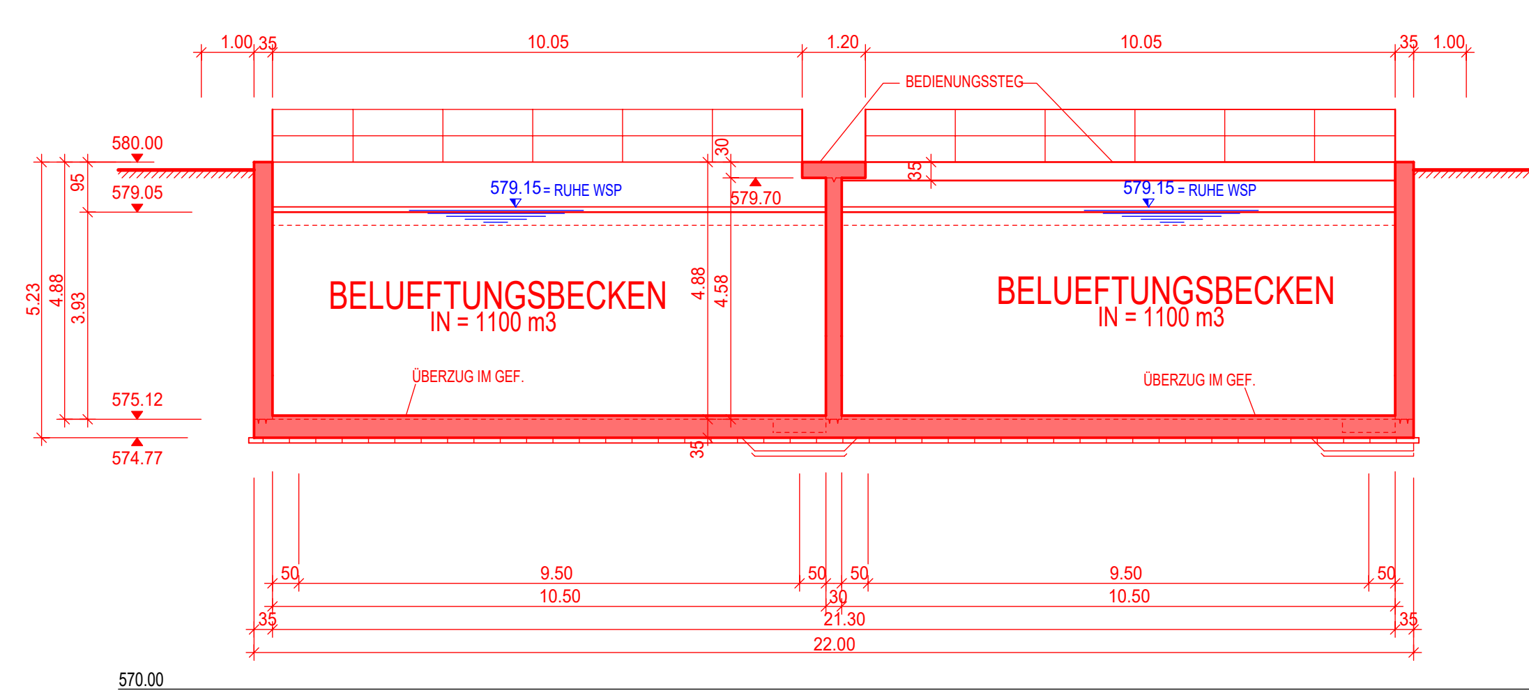
SNCHTT D-D 1 : 100
