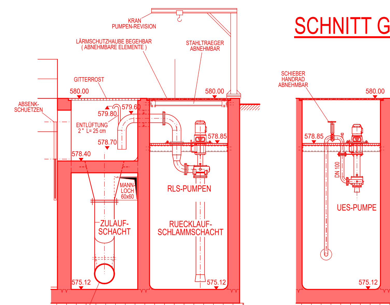
SNCHTT G-G 1 : 50
