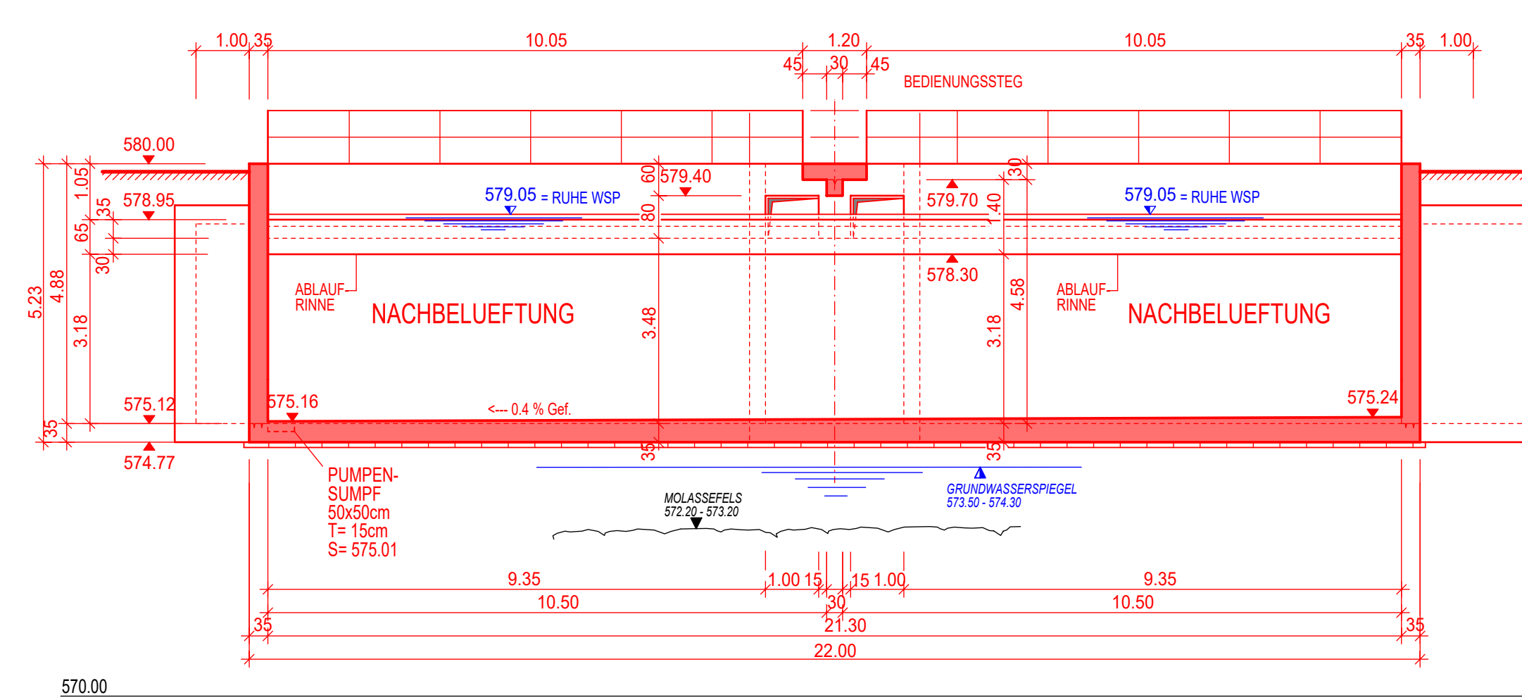
SNCHTT C-C 1 : 100
