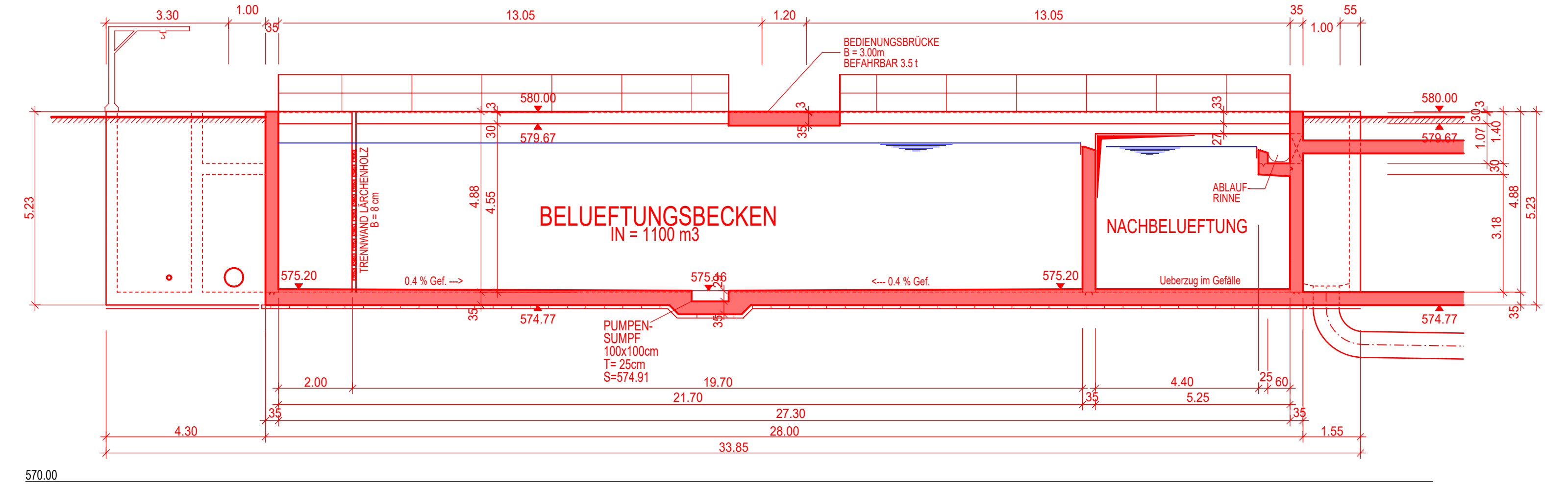
SNCHTT B-B 1 : 100
