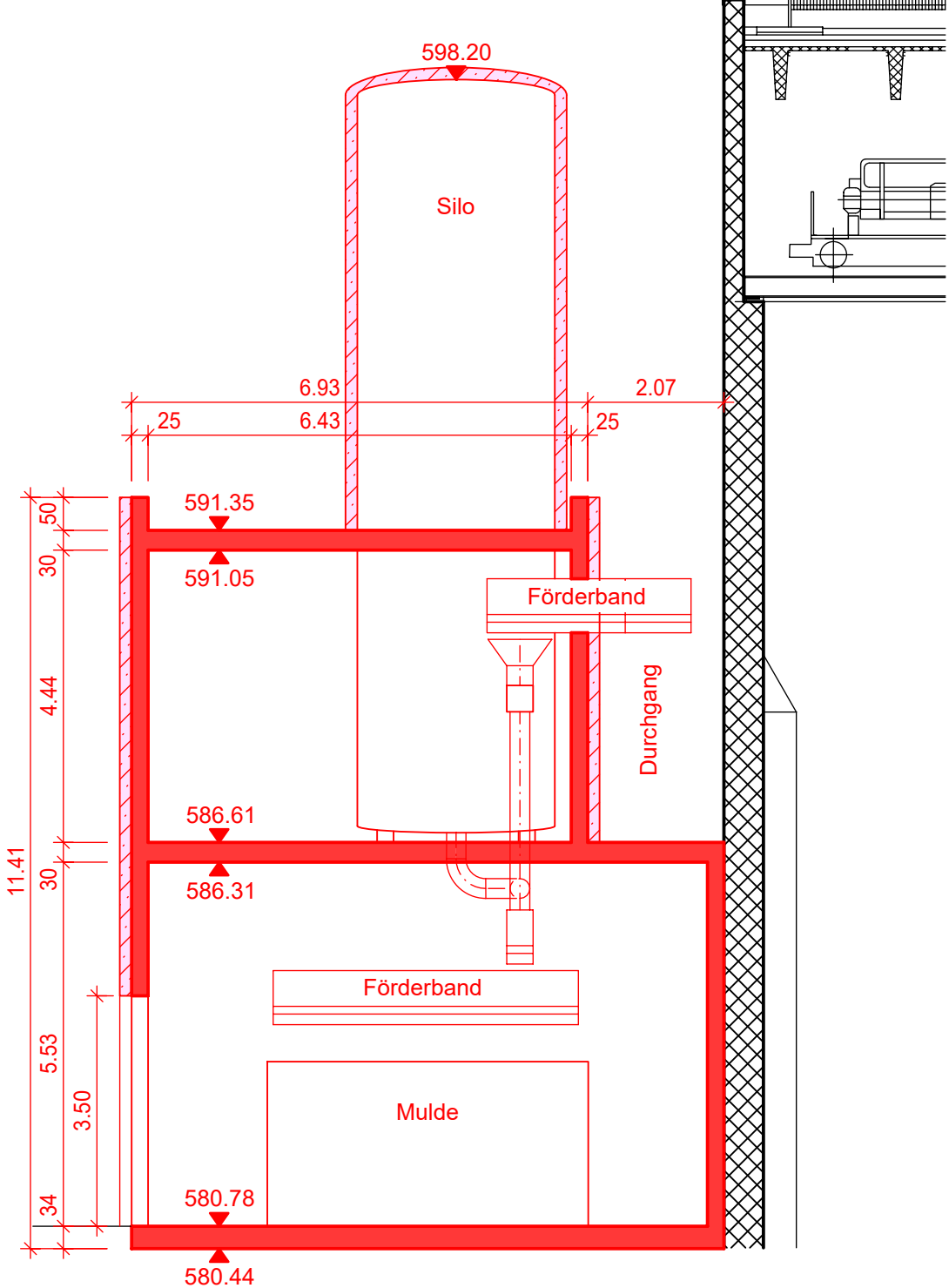
SNITT D-D
