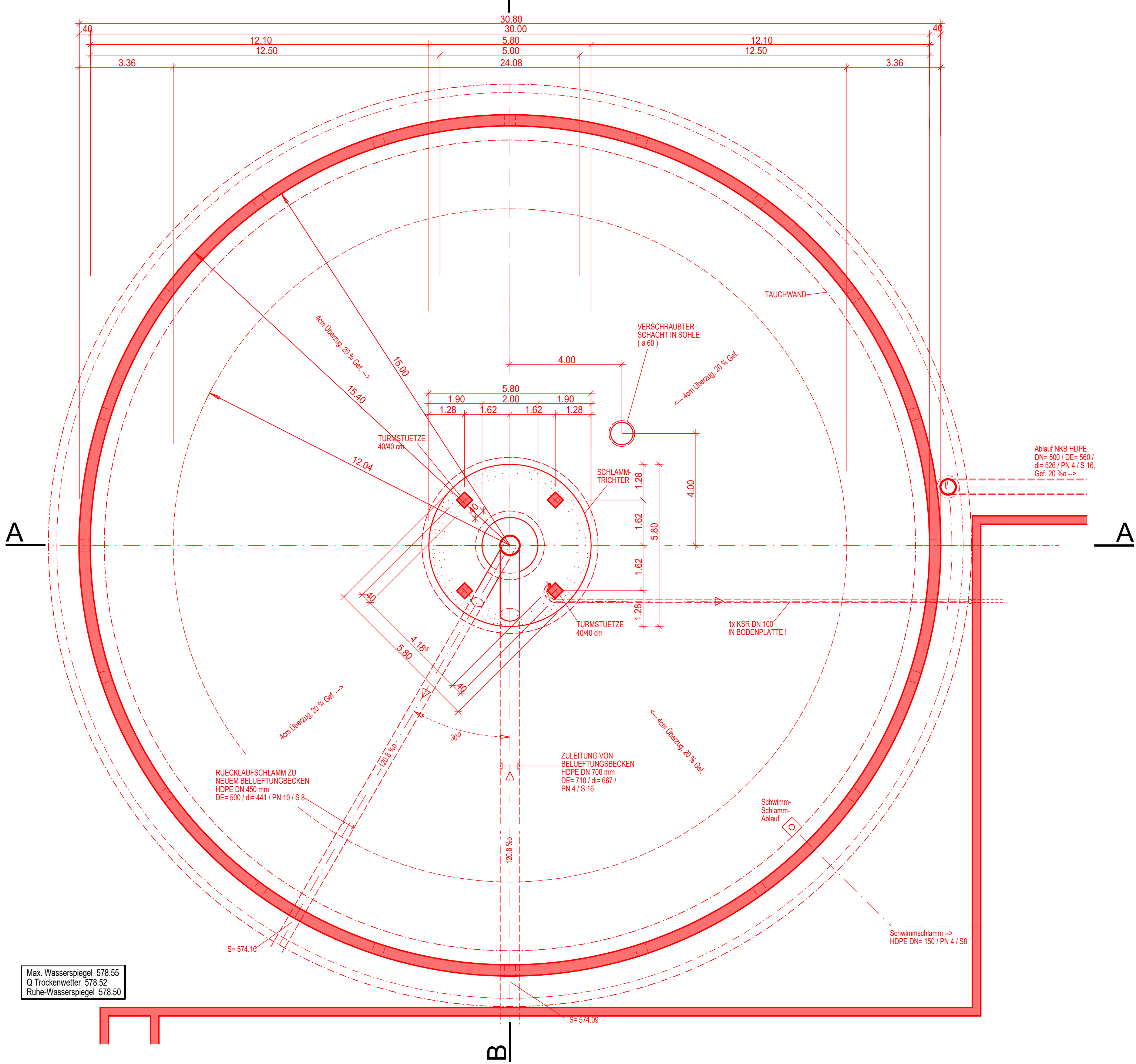
GRUNDRISS 1-1 1 : 100
