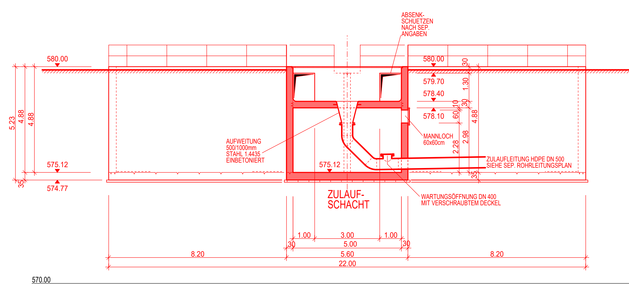
SNCHTT E-E 1 : 100
