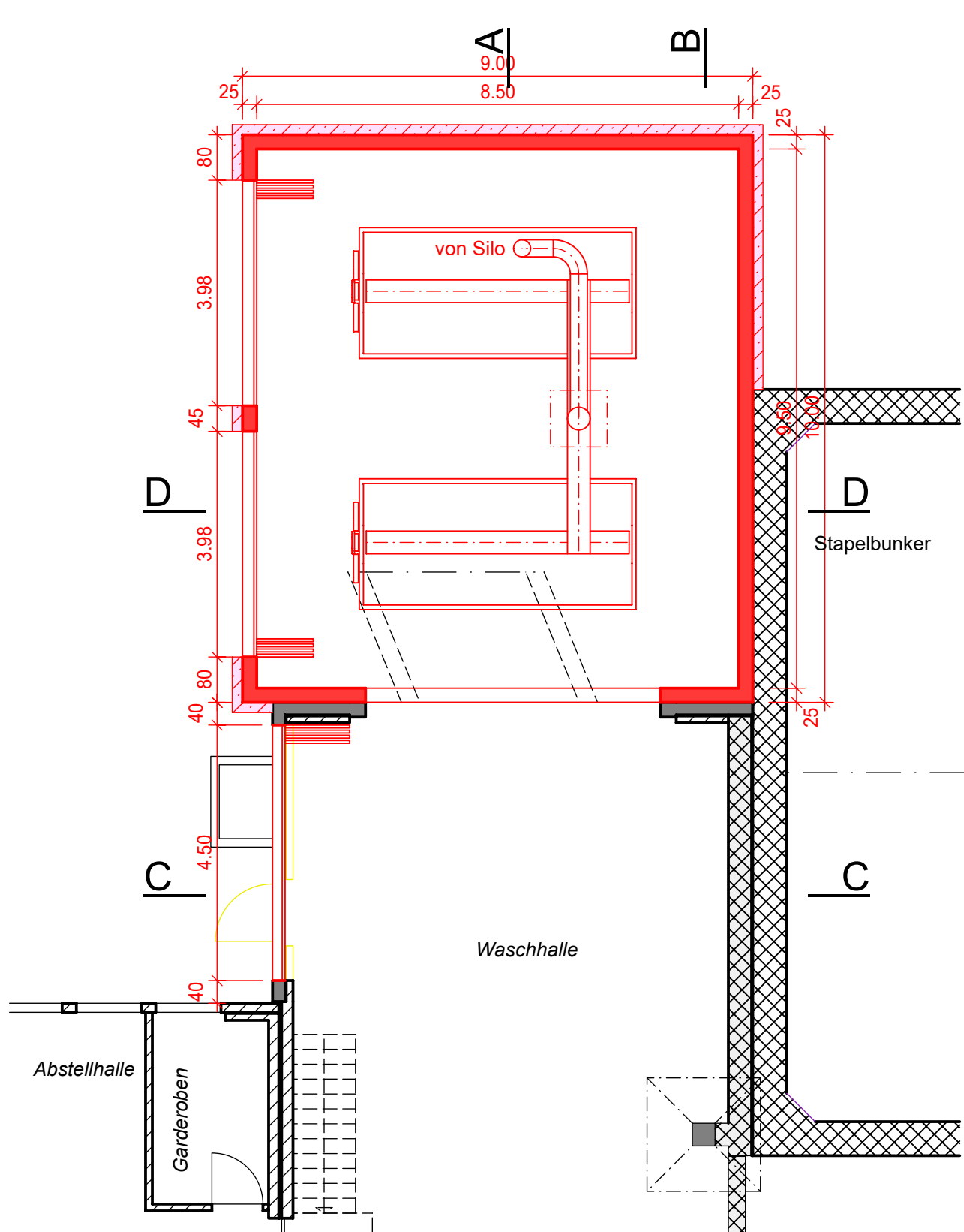
GRUNDRISS EG
