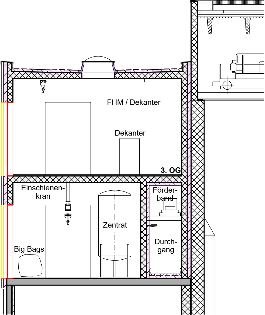
SNITT C-C
