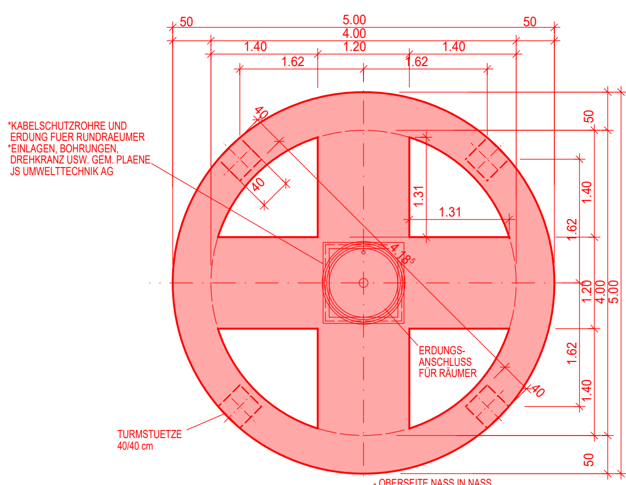
TURM 1 : 50 DRAUFSICHT
