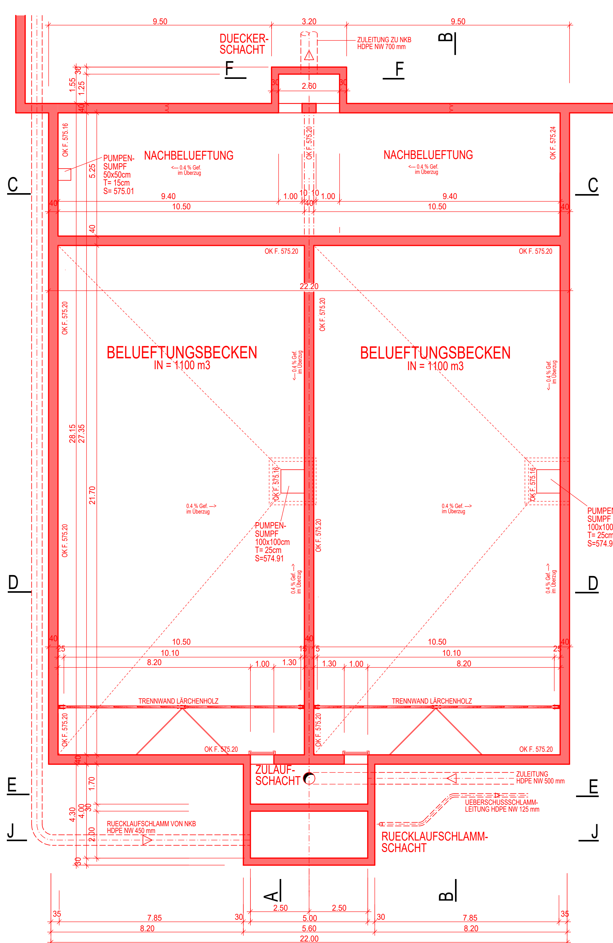
GRUNDRISS WÄNDE 1 : 100
