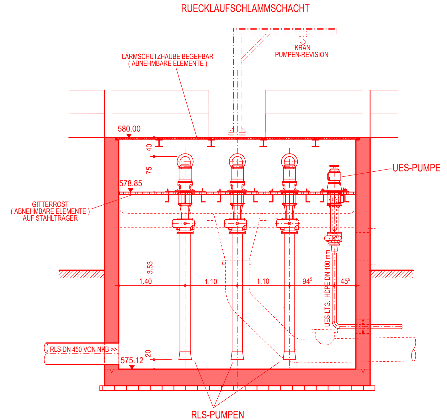
SNCHTT J-J 1 : 50
