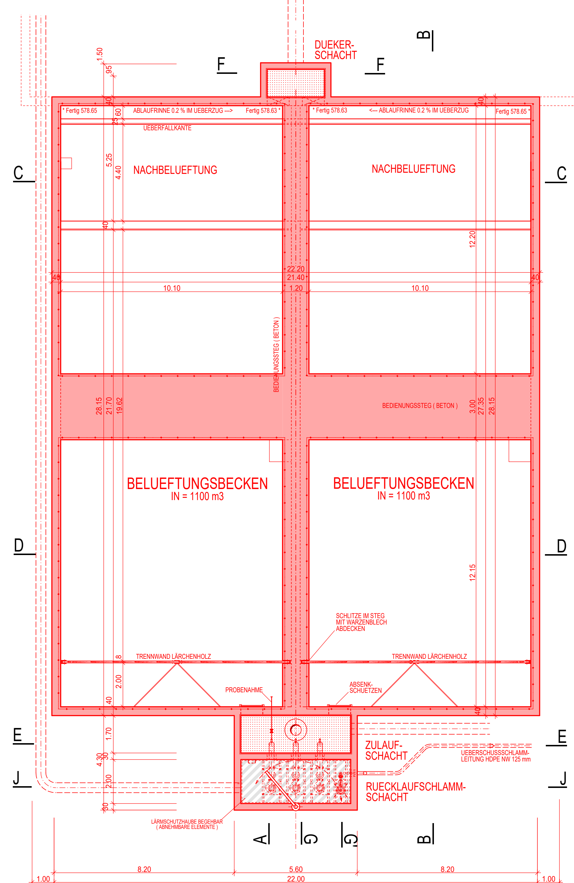
DRAUFSICHT 1 : 100
