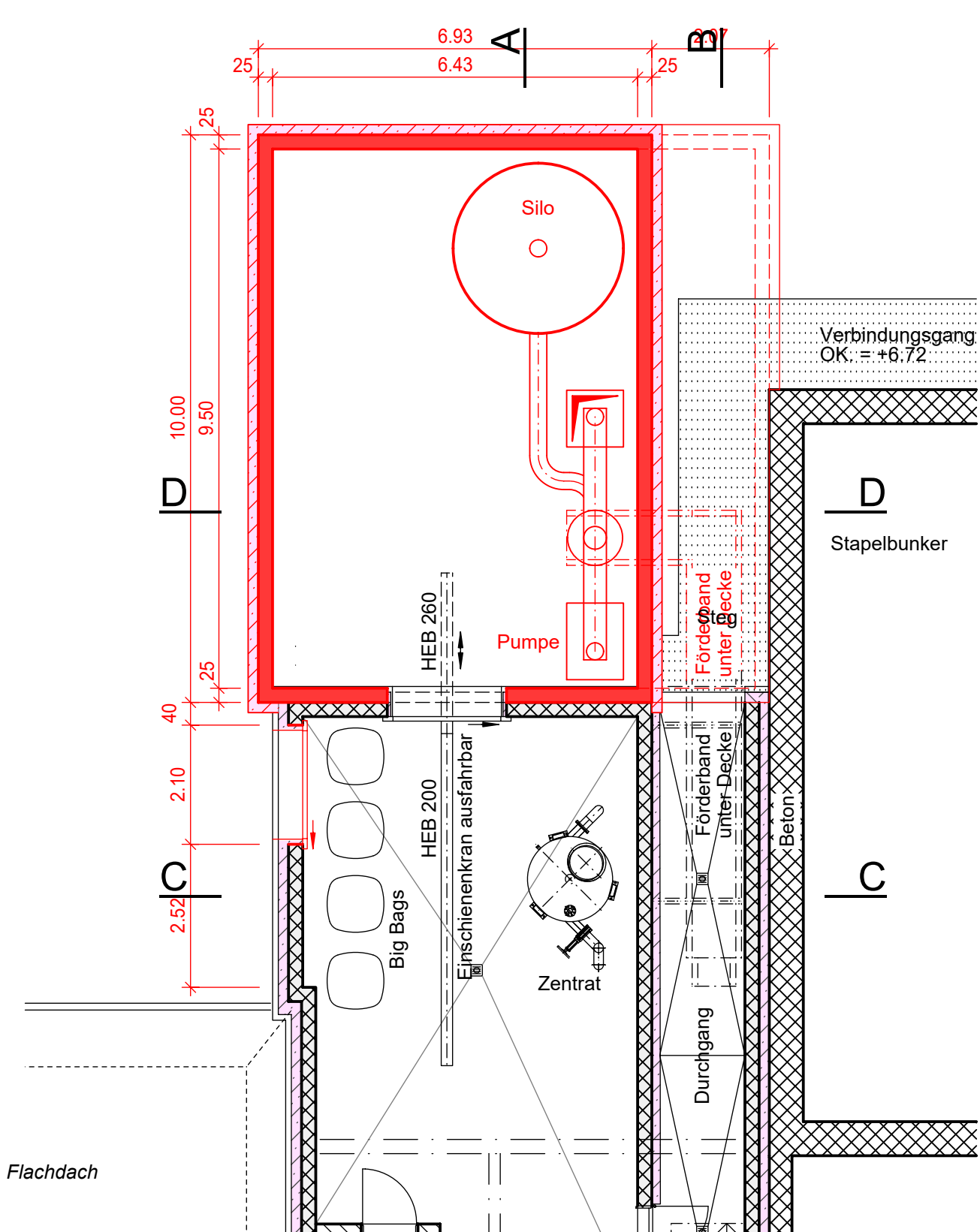
GRUNDRISS 2. OG
