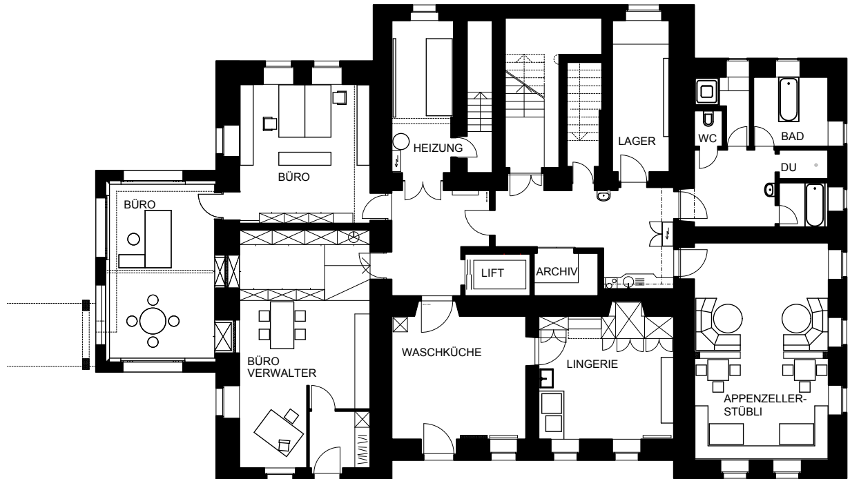
Untergeschoss Bestand
