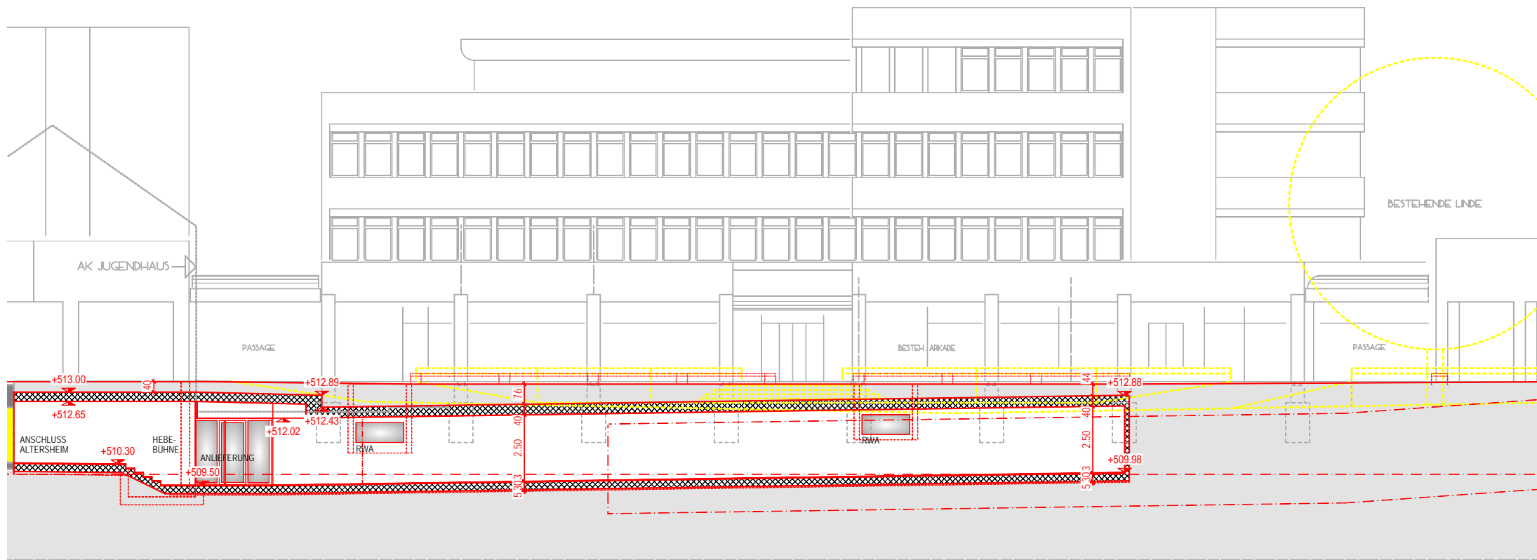
SCHNITT C - C
