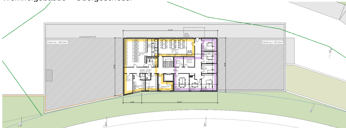
Abbildung 3: Grundriss Obergeschoss
