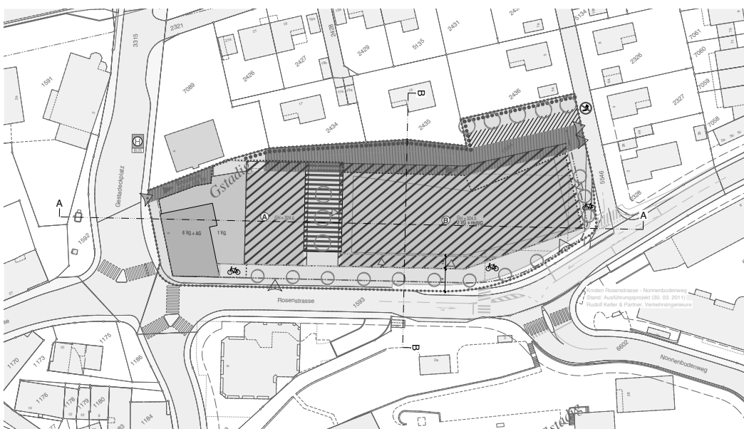
Quartierplan Gstadig
