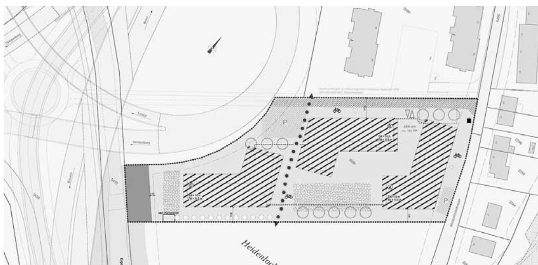
aus: Quartierplan Heidenweid, Situationsplan / Schnittplan 1:500, Kantonale Vorprüfung / öffentliche Mitwirkung
