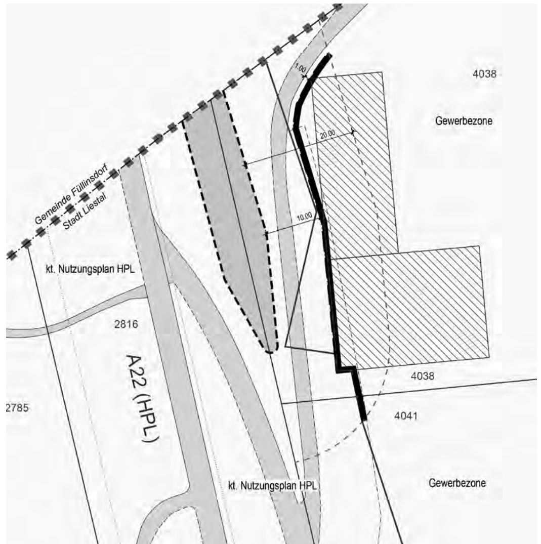
Waldbaulinienplan
