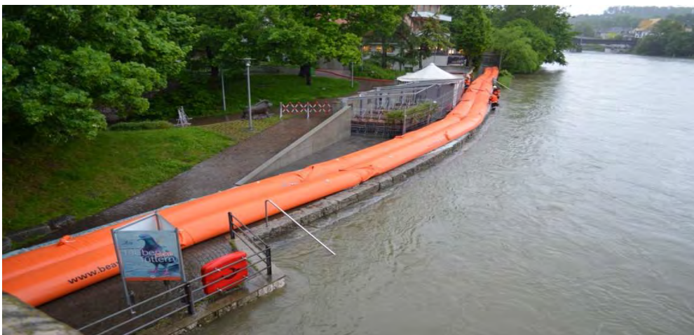
Hochwasser, Bereich Aare Bistro (1.6.13, Hochwasserschutz mittels Beaver-Technik)
