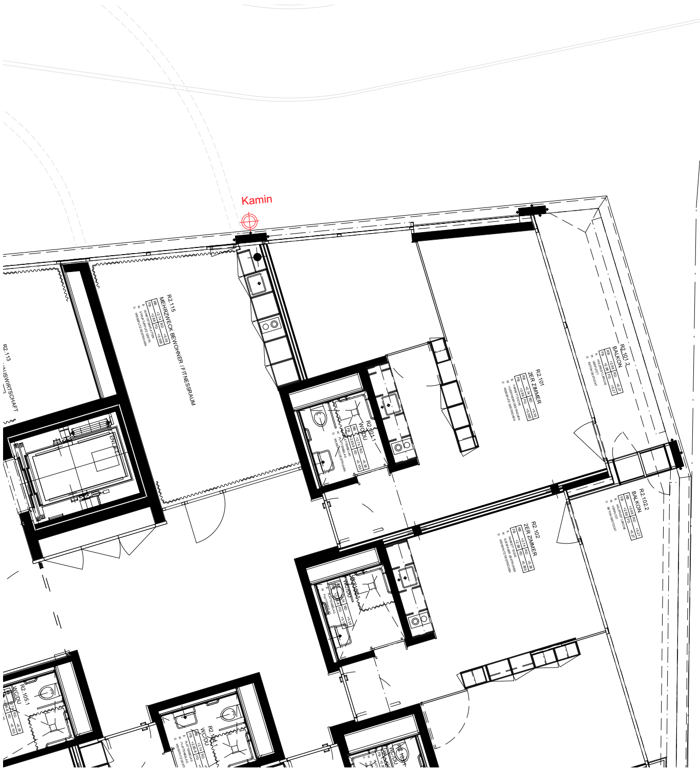
Normalgeschoss
