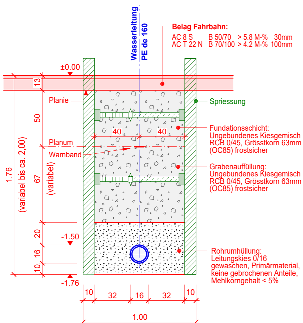
2 - 2 Normalprofil Graben Wasser Föhliweg
