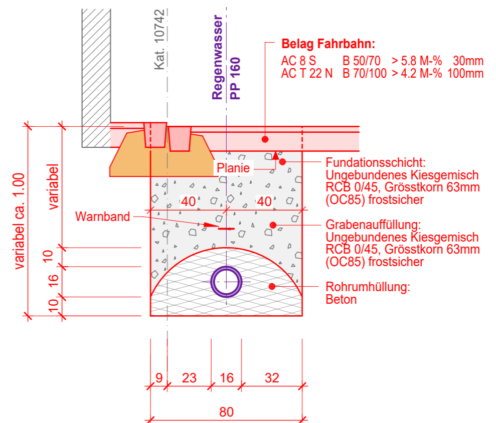
3 - 3 Normalprofil Graben Regenwasser Föhliweg
