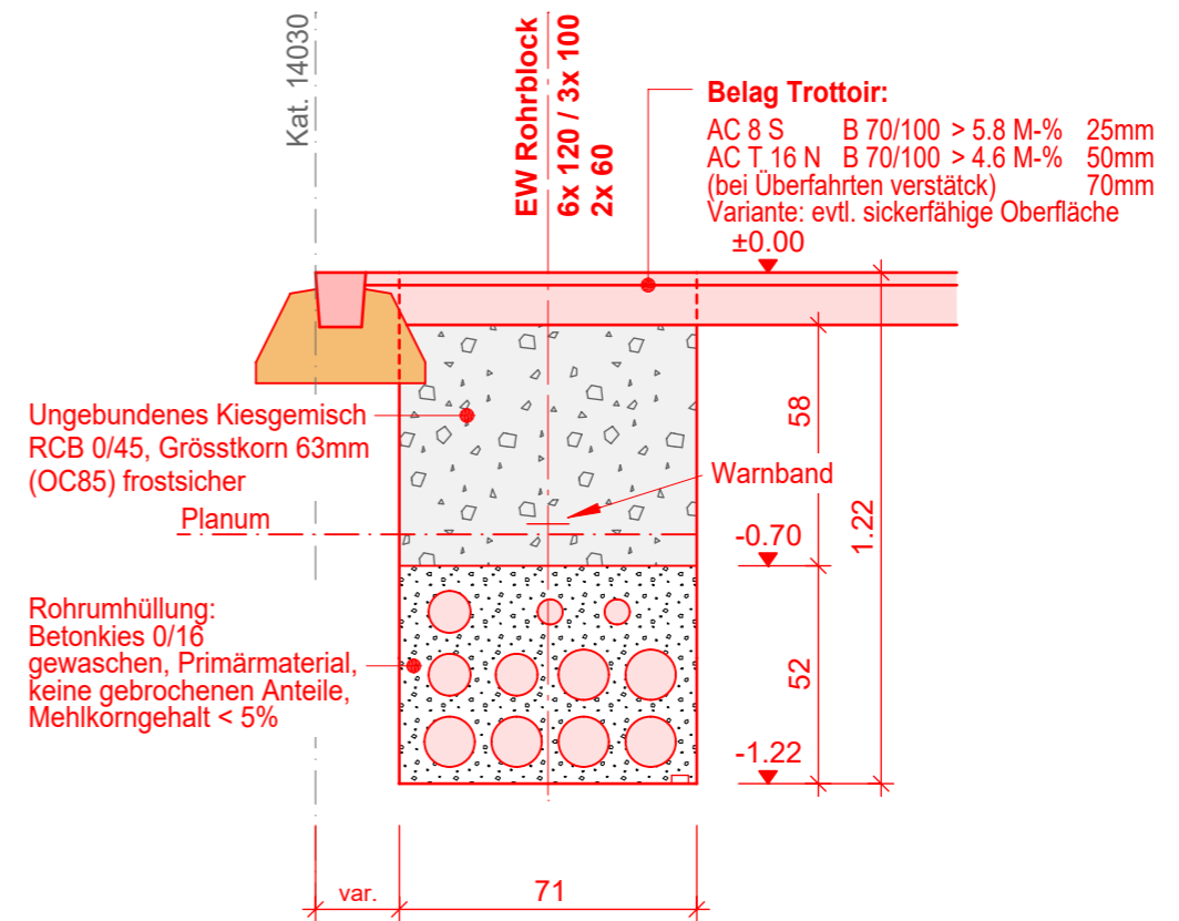
1 - 1 Normalprofil Graben EW Föhliweg
