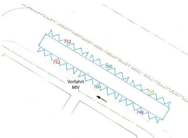
Abbildung 23: V3: Mittelperron (Flieskanten) – Bsp. Bahnhof Uznach
