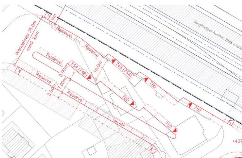
Abbildung 31: Sägezahn - Option mit zweiter Fahrgasse (zusätzliche Reservehaltetellen)
