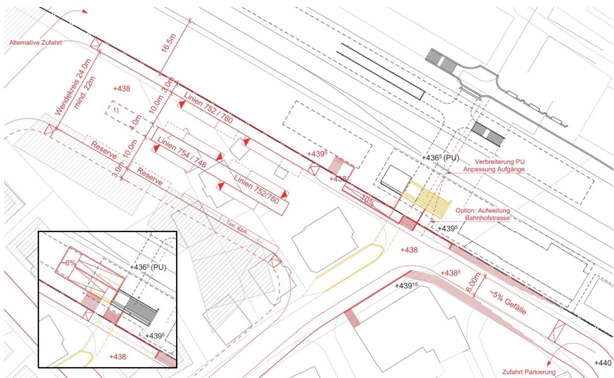
Abbildung 38: Bushof mit reduzierter Platzabsenkung – Prinzipskizze (Basis: Fliesskanten parallel)
