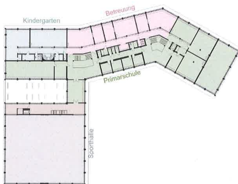
Grundriss 1. Obergeschoss
