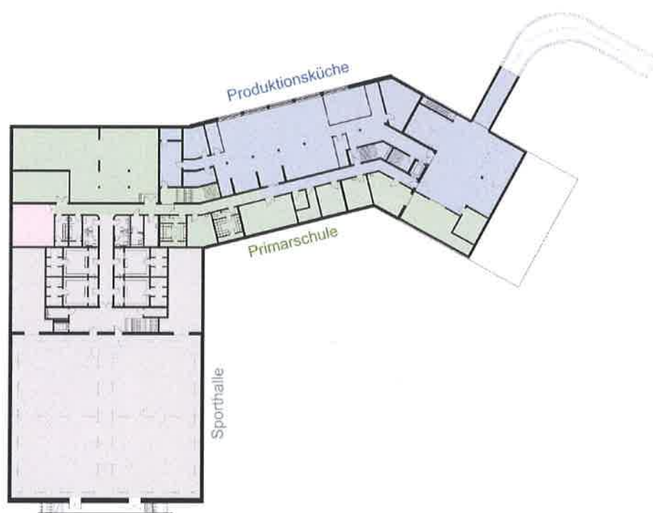
Grundriss Untergeschoss
