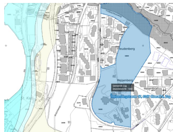
Abbildung 5 Grundwasserkarte, Zugmap, 8.3.2023
