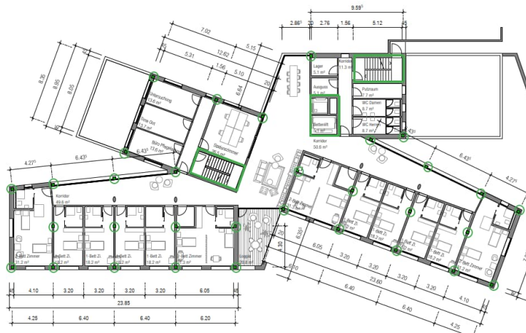
Abbildung 14 Stützenraster Haus ND gemäss Richtprojekt von Diener & Diener Architekten
