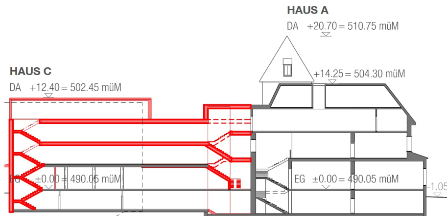
Abbildung 16 Schnitt durch Haus A & C mit Erhalt bestehender Bausubstanz, Quelle: Richtprojekt von Diener & Diener Architekten
