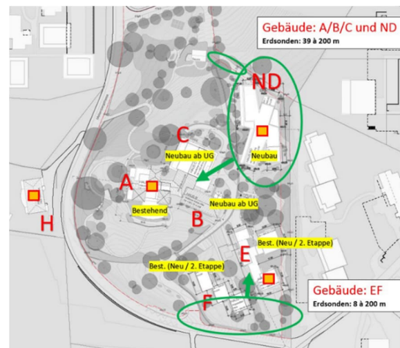
Abbildung 3 Erdwärmesonden
