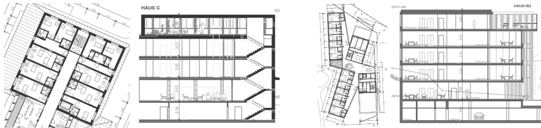
Abbildung 12 1. OG und Schnitt Haus C (links) & 1. OG und Schnitt Haus ND (rechts) gemäss Richtprojekt von Diener & Diener Architekten
