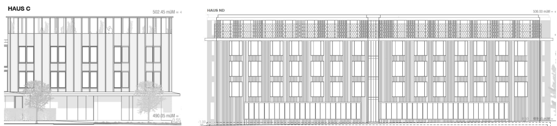
Abbildung 15 Ansichten Haus C (links) und ND (rechts) gemäss Richtprojekt von Diener & Diener Architekten
