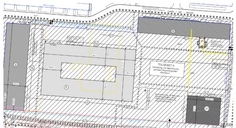
Abb. 2: Bebauungsplan städtischer Grund vor dem Stadthaus Zug. Die gelbe Markierung zeigt die Unterkellerung für die Tiefgarage. Detailansicht inklusive Legende: Foyer 7001 (zg.ch)
