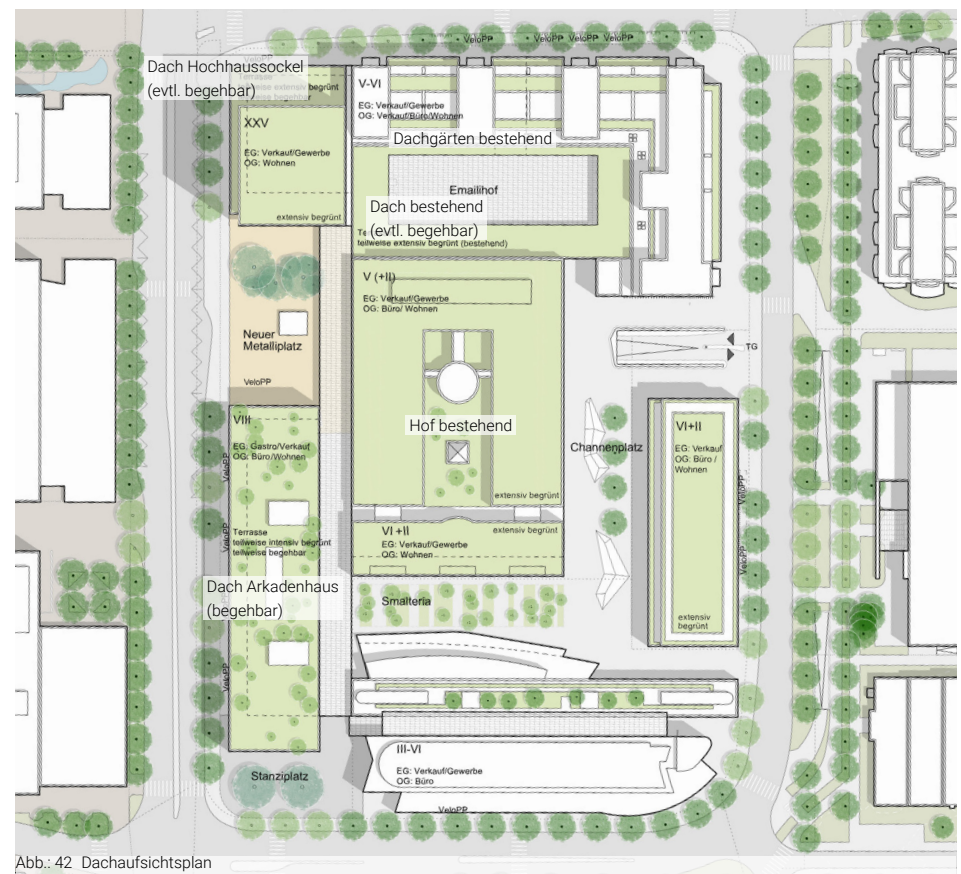
Abb.: 42 Dachaufsichtsplan
