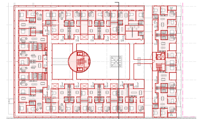
Abb.: 22 Grundriss OG zentraler Bau (Wohnen)
