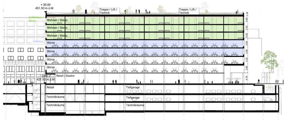
Abb.: 17 Schnitt Arkadenhaus
