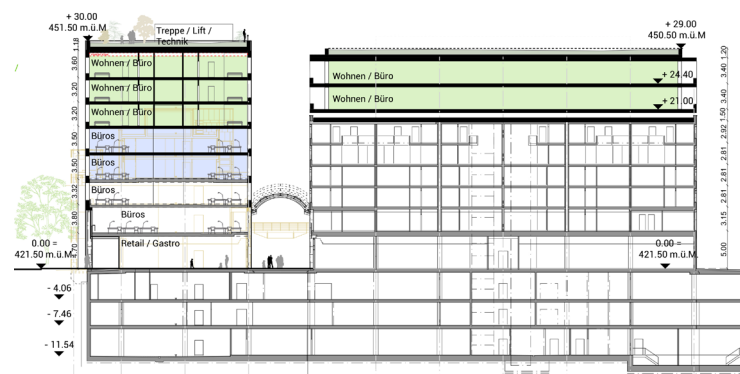
Abb.: 21 Schnitt zentraler Bau
