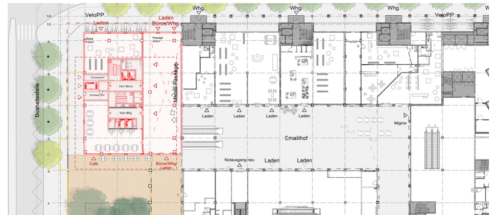
Abb.: 16 Grundriss EG Hochhaus
