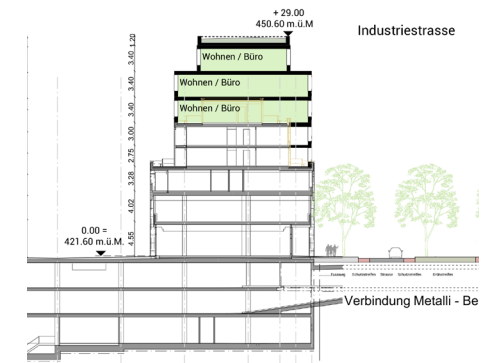
Abb.: 23 Schnitt Bau Ost
