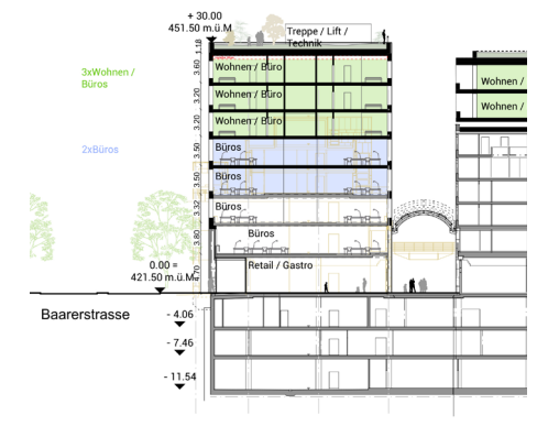
Abb.: 19 Schnitt Arkadenhaus
