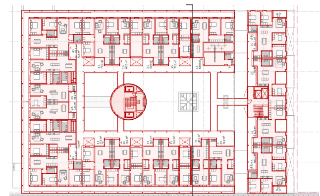
Abb.: 22 Grundriss OG zentraler Bau (Wohnen)
