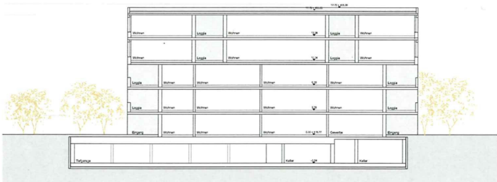
Schnitt B-B'
