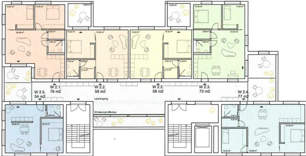
OG2
