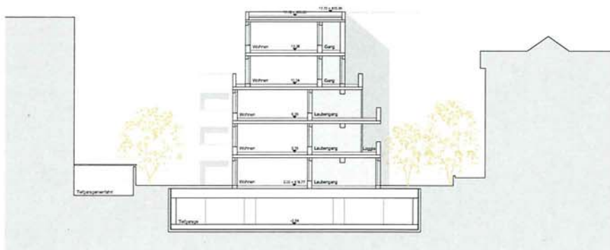
Schnitt A-A'
