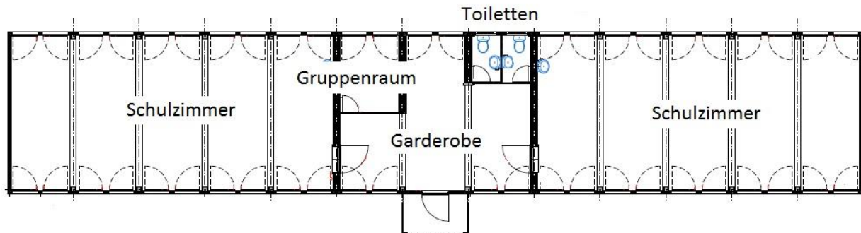
Bild 2: Grundriss Schulraumprovisorium
