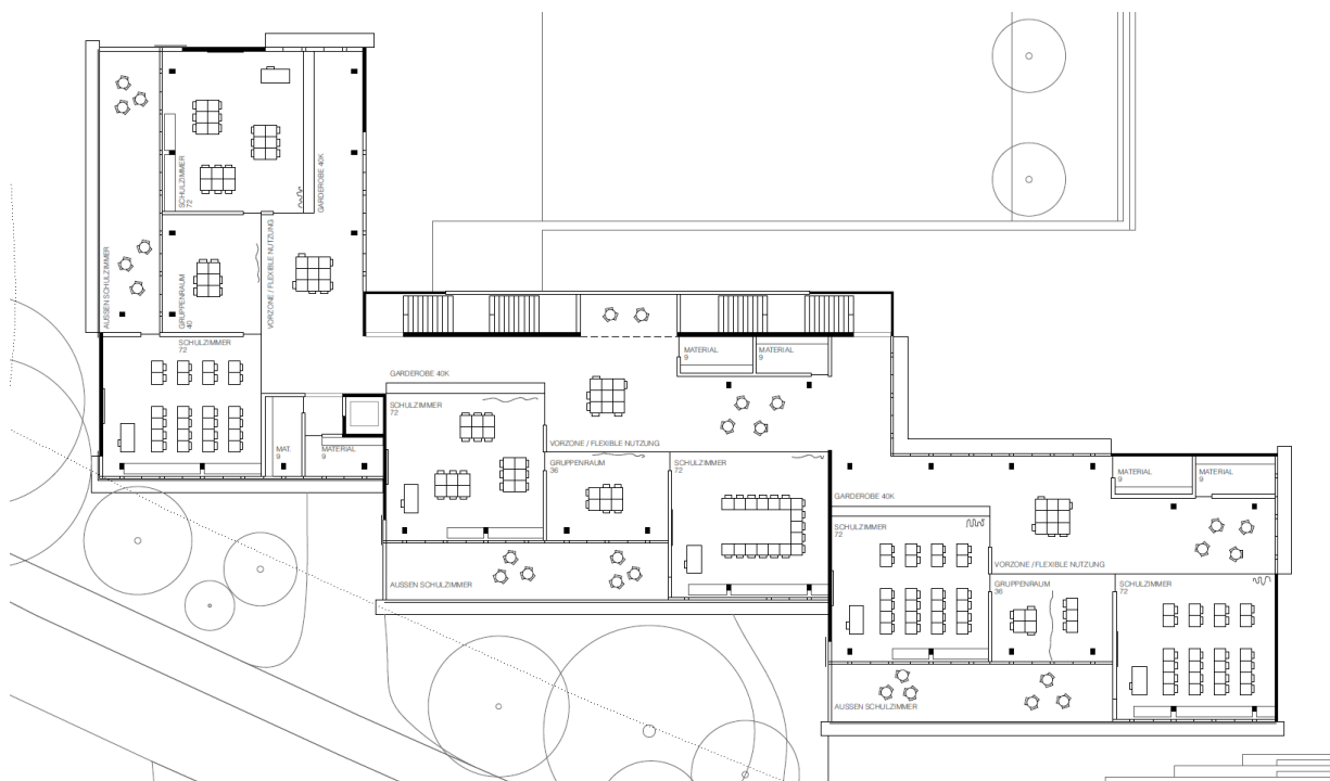
Bild 6: Grundriss Obergeschoss des Siegerprojekts BILL
