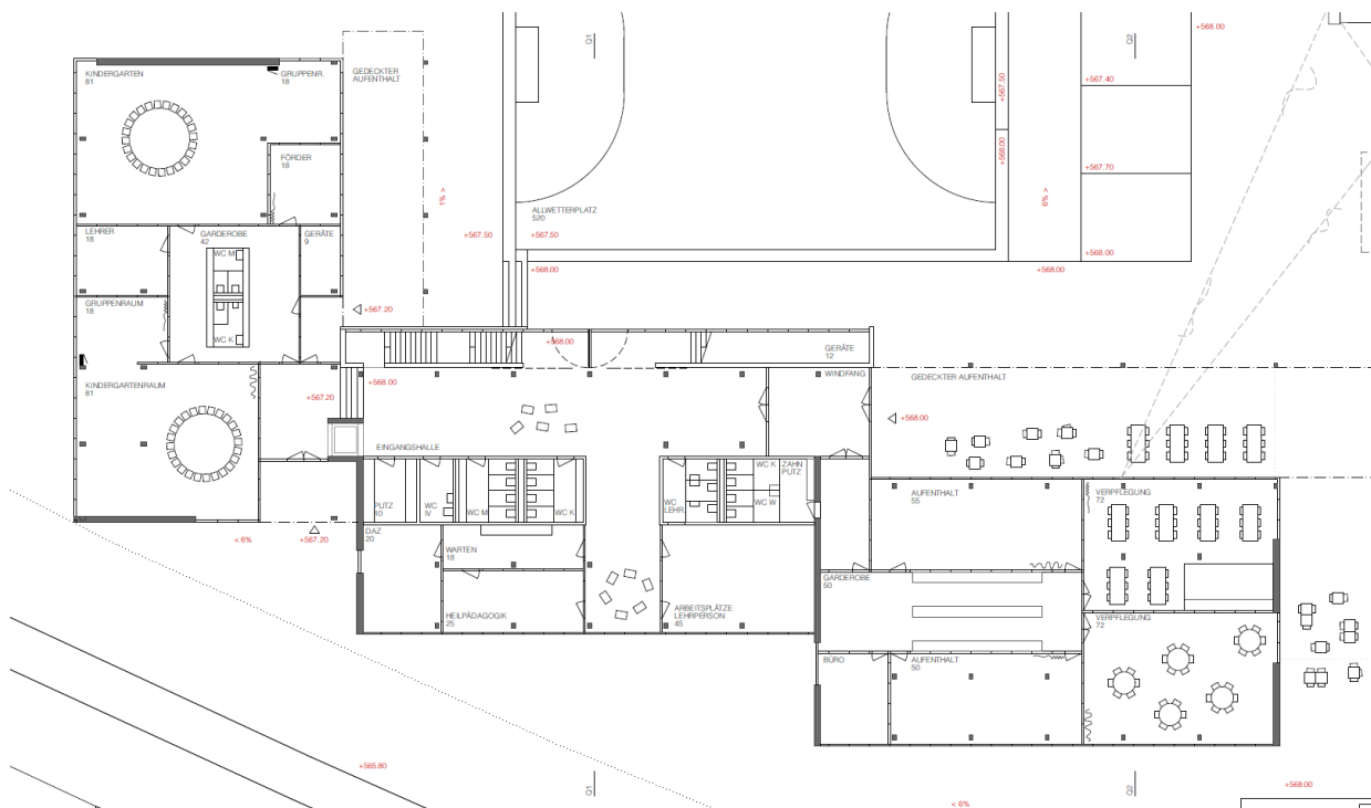
Bild 9: Grundriss Erdgeschoss des überarbeiteten Siegerprojekts
