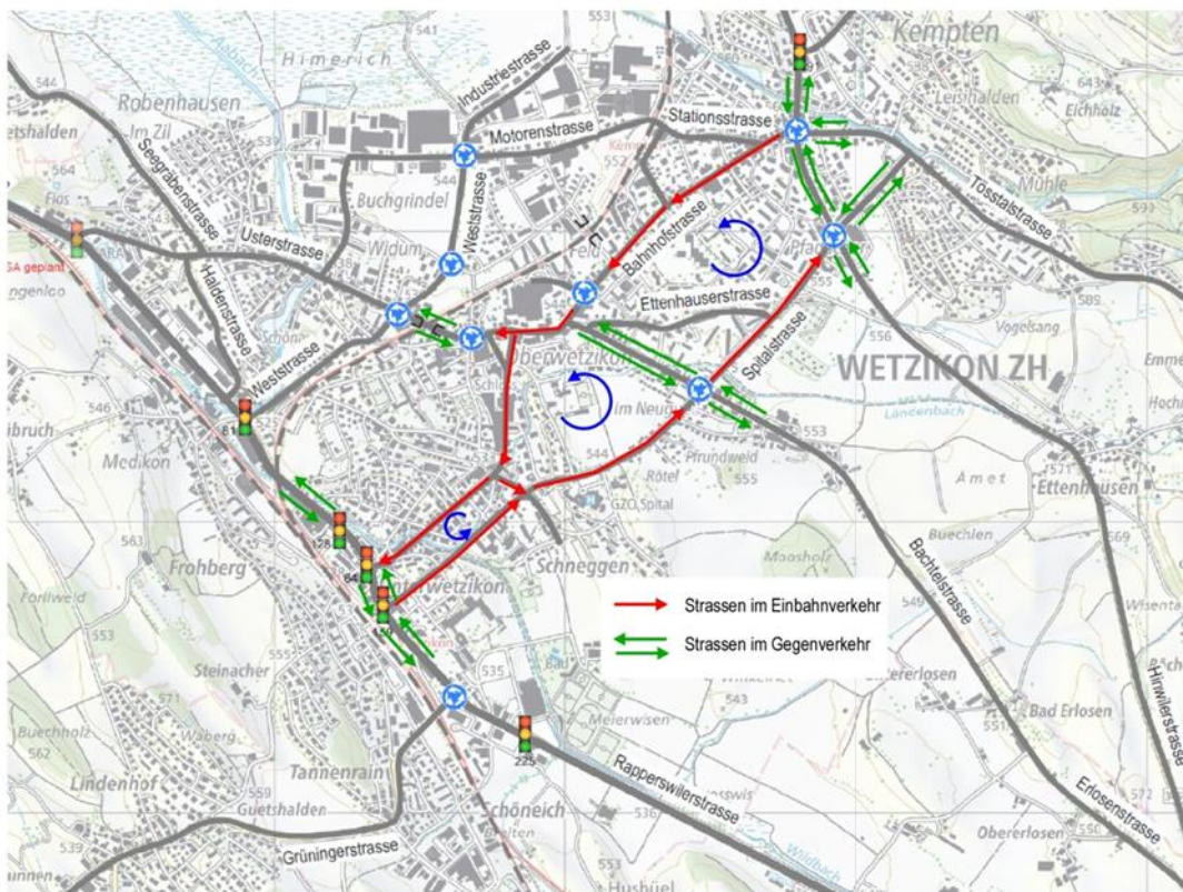
Abb. 5: Untersuchtes Einbahnsystem
