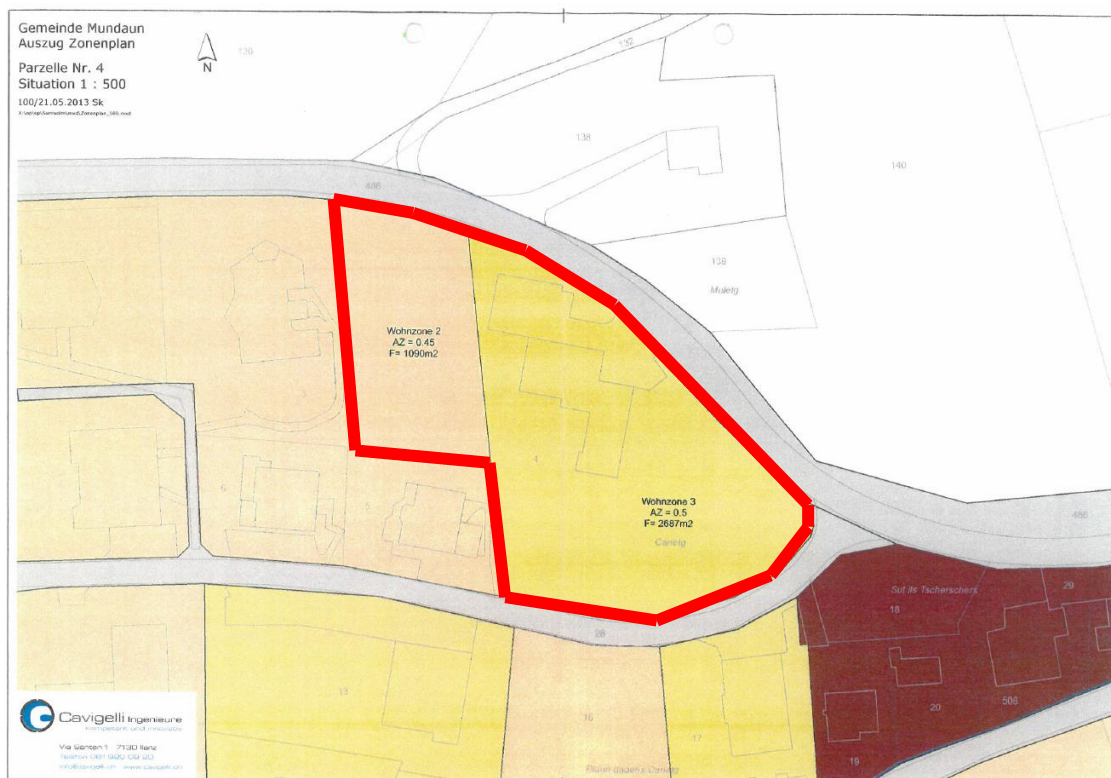
Bild Situationsplan: Wohnzone 2 mit 1'090m 2 , Wohnzone 3 mit 2'687m 2 = Total 3'777m 2
