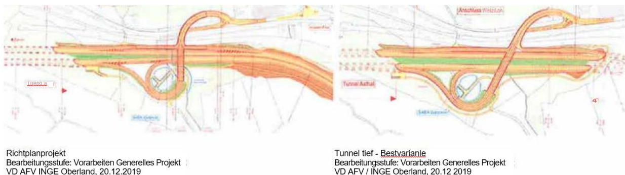
Abb. 1: Autobahnanschluss Wetzikon (Varianten "Richtplanprojekt" und "Tunnel tief")
