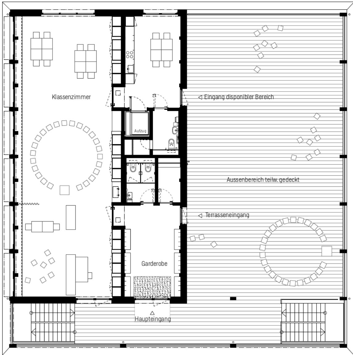
Bild 7: Grundriss Obergeschoss Dreifachkindergarten Kempton
