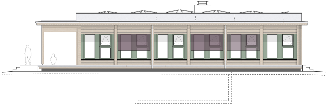
Bild 14: Ostfassade Zweifachkindergarten Goldbühl und Egg
