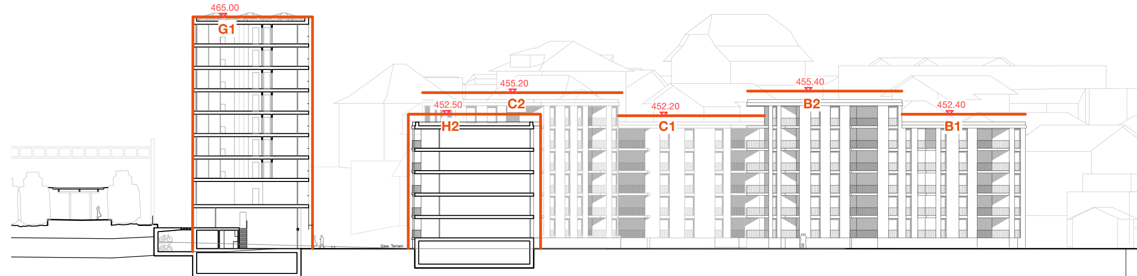
Schnitt A-A 1:500
